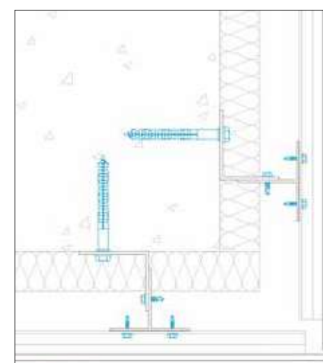
Angolo Esterno External angle Angle sortant Aussenecke Esquina Внешний угол
