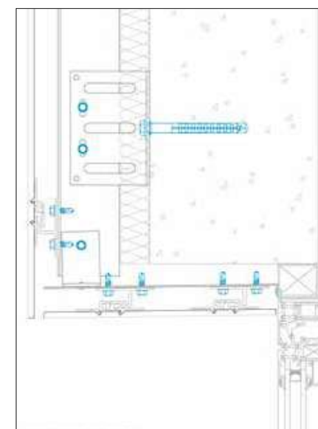
Sezione verticale rivolto finestra Vertical section Section verticale Fensterlaibung Vertikalschnitt Sección vertical recerco de la ventana Вертикальное сечение откос окна
