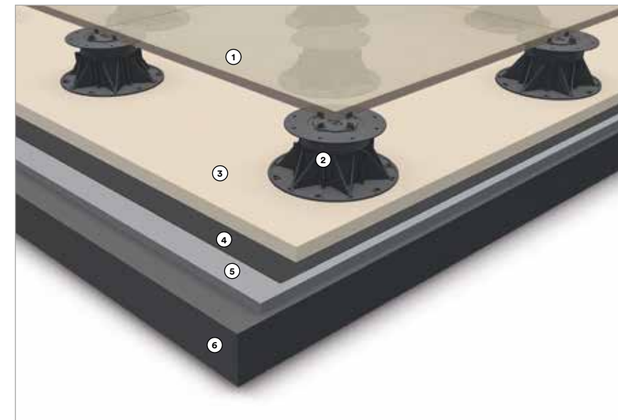
Possibili configurazioni dei supporti • Possible pedestal layouts • Mögliche Konfigurationen der Stelzlager • Configurations possibles des supports • Posibles configuraciones de los soportes • Возможные схемы расположения опор
