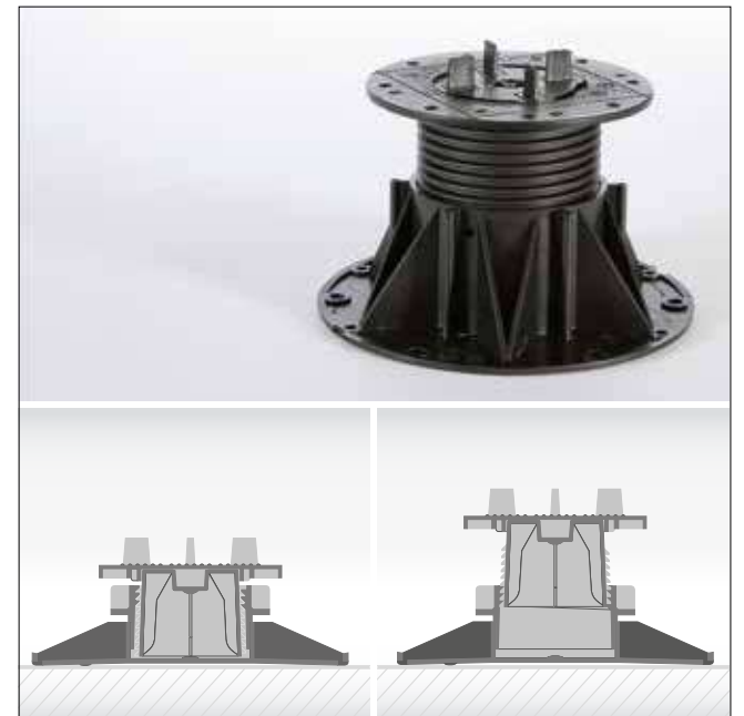
Supporti regolabili • Adjustable pedestals • Supports réglables • Verstellbare stützlagern • Soportes regulables • Регулируемые опоры
