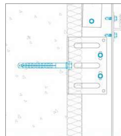
Sezione verticale Vertical section Section verticale Vertikalschnitt Sección vertical Вертикальное сечение
